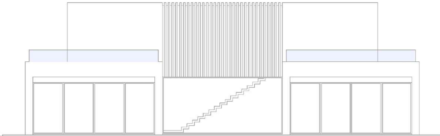
Prospetto Lato Mare
