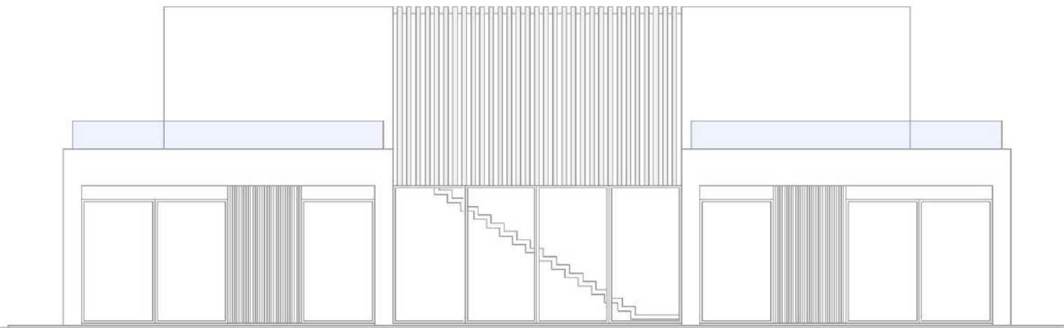
Prospetto Lato Monti
